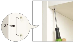
パーツを取り付けるシステム穴は32mm間隔
